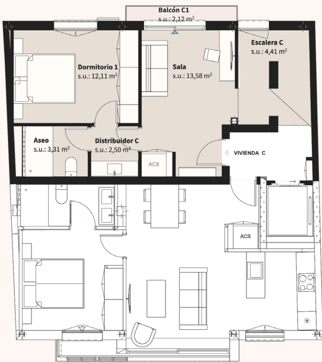
Planta Piso Segunda. Vivienda C.
