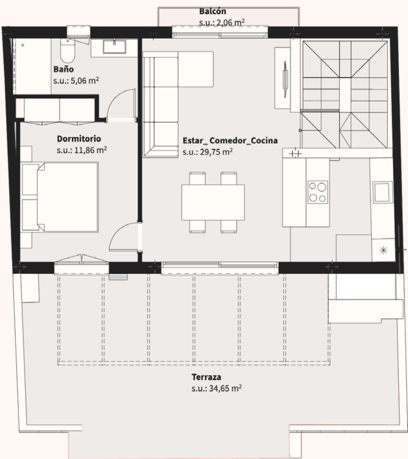
Planta Piso Tercera. Vivienda C.
